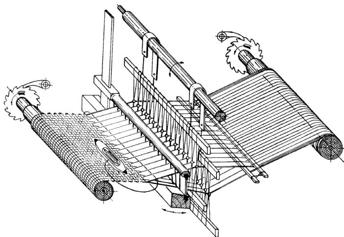
funkční část ručního tkalcovského stavu
